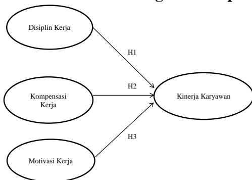
Gambar 1. Kerangka Konseptual
